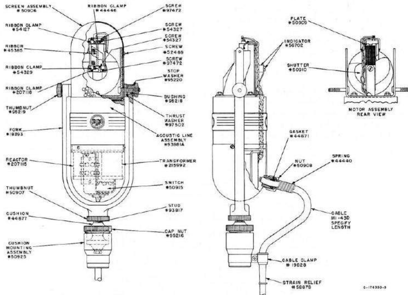
Figura 30 – Imagem da estrutura interna do Microfone RCA TYPE77DX.
